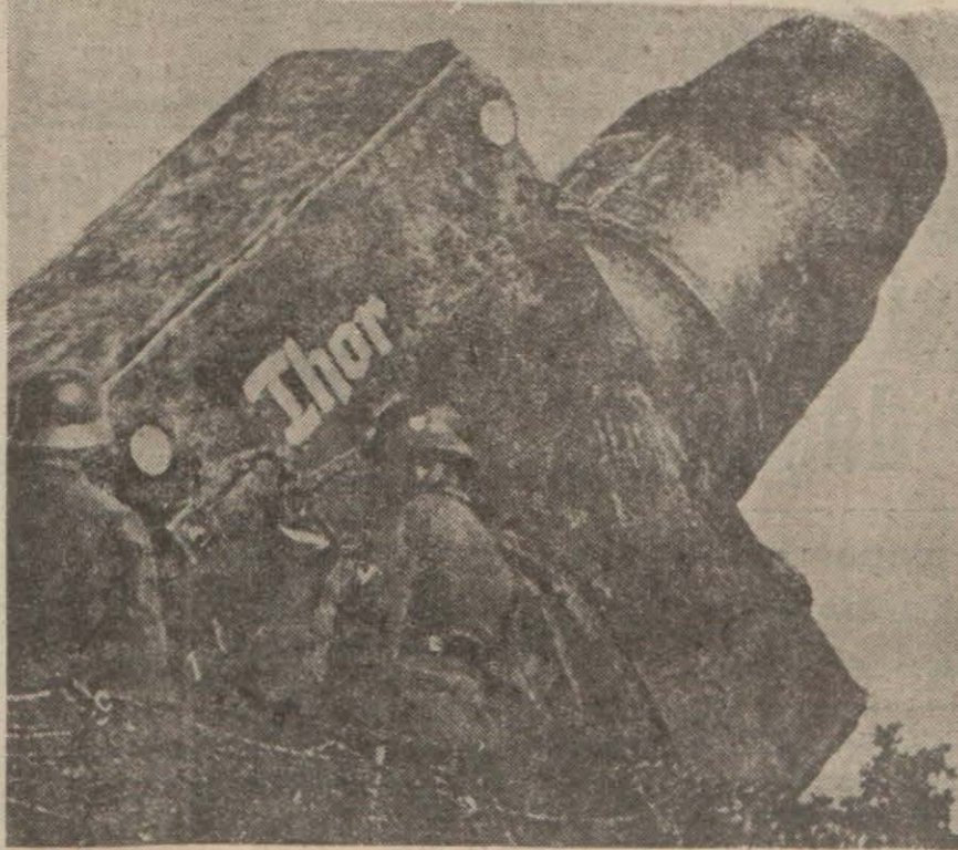
Sivastopol'un bombardmanı esnasında kullanılan ve «Thor» tesmiye edilen son model bir Alman ağır topu
